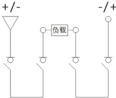
接线图 1 4P 外形 C型接线方式
